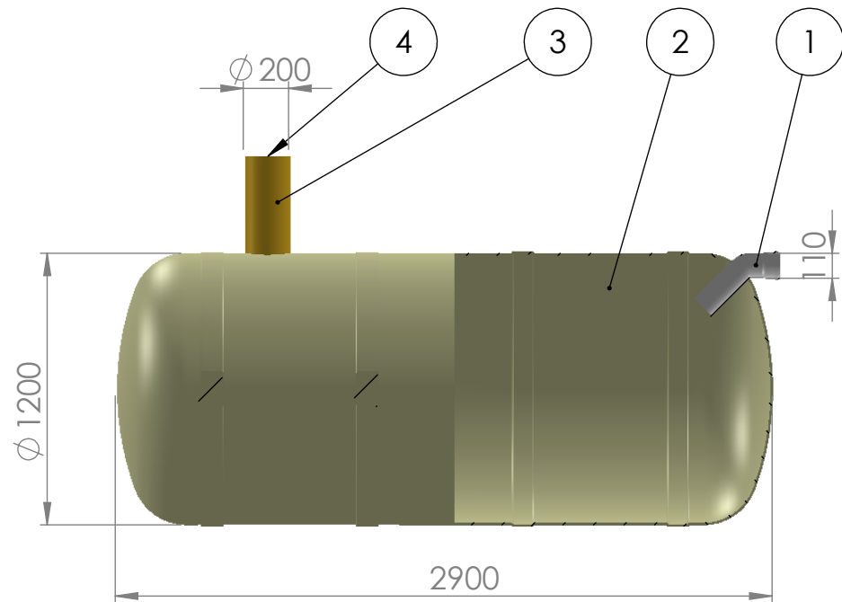
SECTION A-A SCALE 1 : 30
